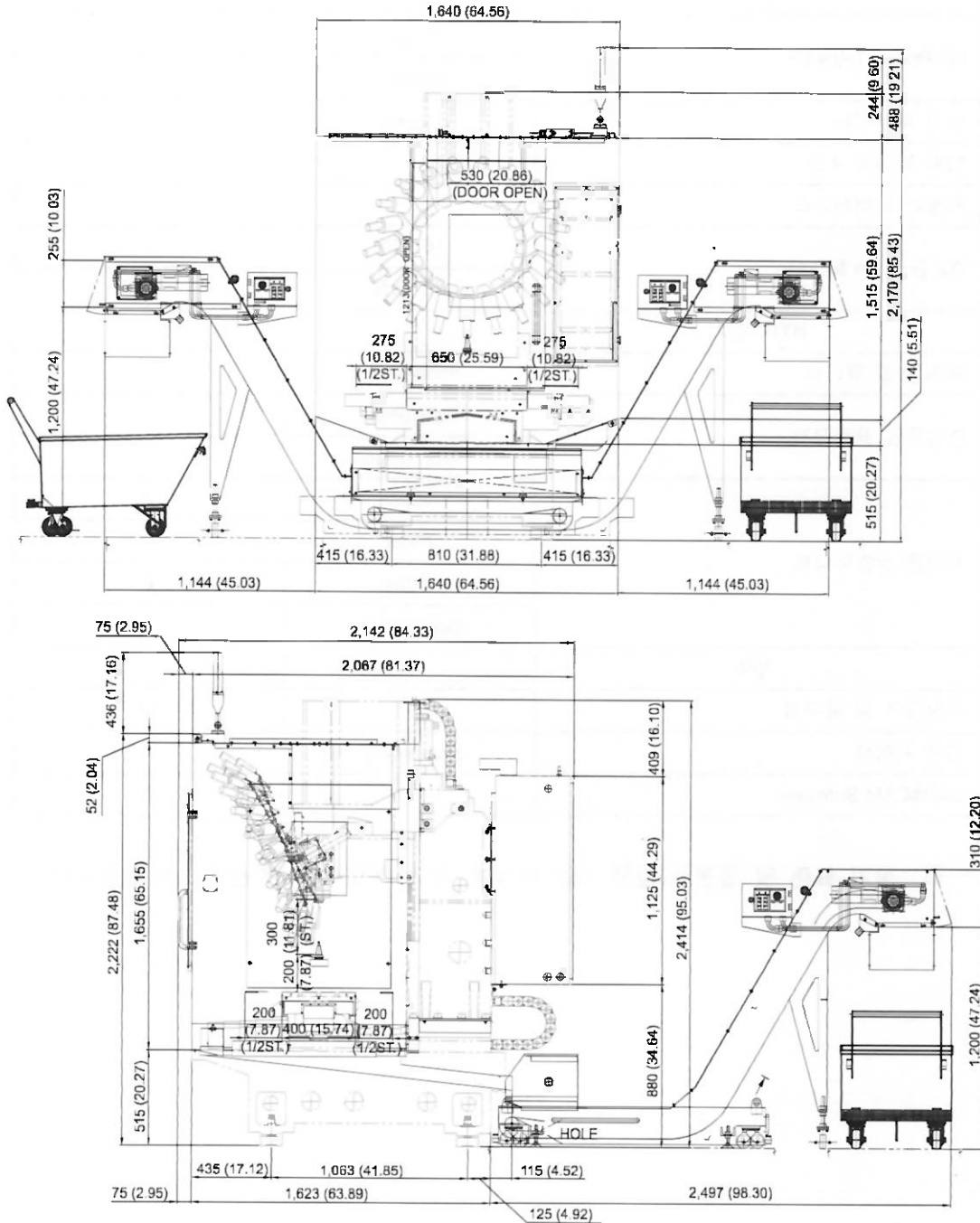
그림 1.4 외형 치수도 (단위: mm (inch))
